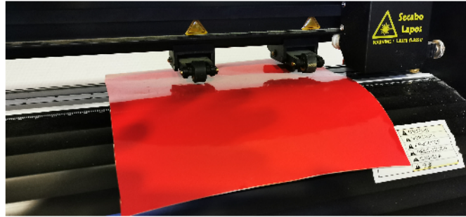
3. Folie einfädeln und ausrichten. PLatzierung der Andruckrollen justieren. Mindestens 2 Rollen.
